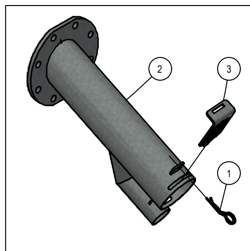
Ballenvanger (optie)
